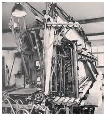
Automatenschiffchenstickmaschine. (HistAL, Fotoarchiv, A I 23)
